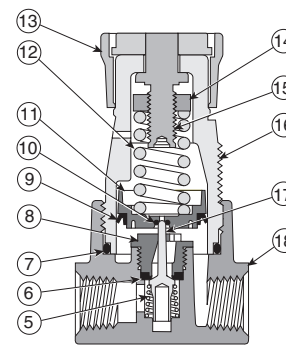
FIGURE 2 – Régulateur miniature, sans équilibre, avec dispositif d'évacuation montré
