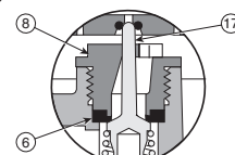
FIGURA 3: Detalle del sello del obturador
